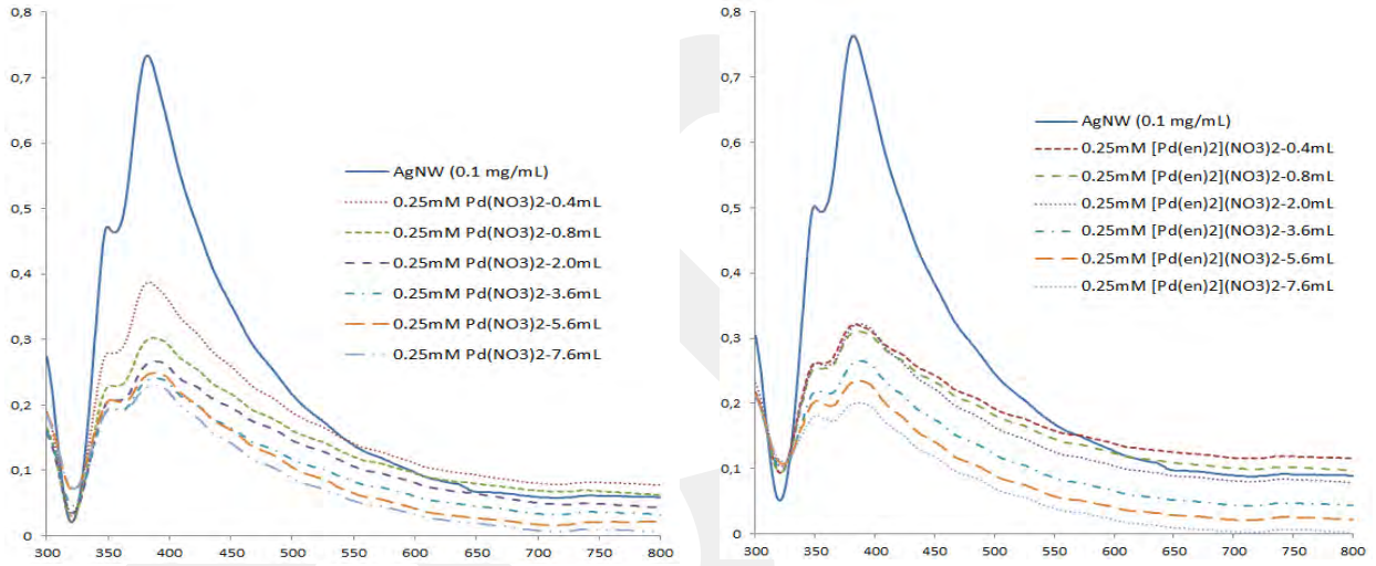
Şekil 46. Sulu çözelti içerisinde Ad@Pd nanotellerle ait UV-görünür bölge spektrumları. Ag nanotel için SPR pik şiddetindeki azalma ve hafif kızıla kayma görülmektedir.
