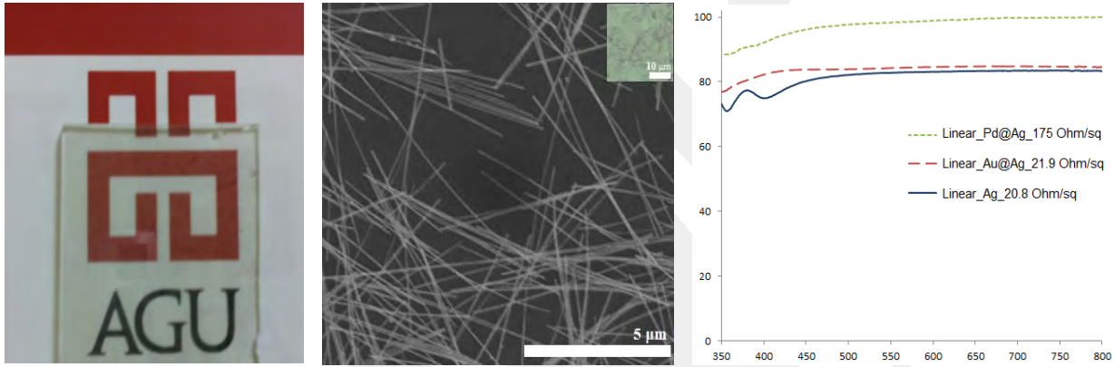
Şekil 45. Polikarbonat substrat üzerinde arka zemini gösteren Ag@Pd nanotel filmine ait fotoğraf (solda). Ag@Pd nanotel filmlere ait SEM ve ışık mikroskopu (küçük resim) görüntüsü (ortada). Aynı filme ait, ortalama 95% geçirgenlik ve ~1,9% bulanıklık oranı gösteren Uv-görünür bölge spektrumu (sağda). Filmin levha direnci 4-noktalı prob kullanılarak 175 Ohm/sp olarak ölçüldü. Kıyaslamak amacıyla, daha önceki çalışmamızdaki Ag nanotel filme (levha direnci: 21,9 Ohm/sq) ve Ag@Au nanotel filme (levha direnci:20,8 Ohm/sq) ait UV-görünür bölge spektrumu da birlikte çizildi.
