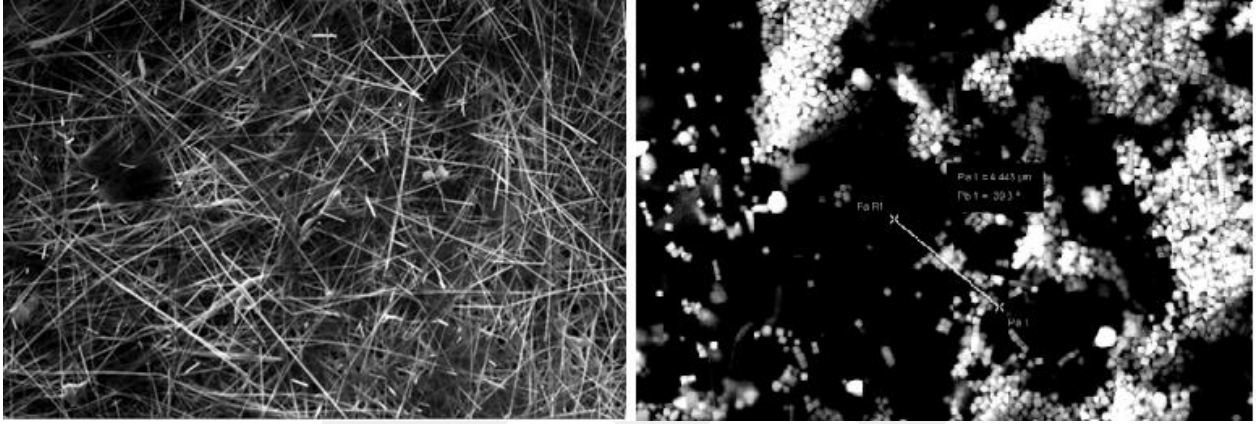
Şekil 48. 185 °C'de 48 saat bekletilen reaktörden elde edilen bakır nanotellere ait SEM görüntüsü (solda), üst katmana ait SEM görüntüsü (sağda).
