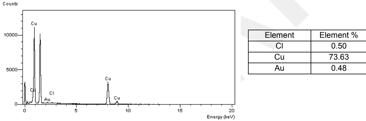
Şekil 21. \text{HAuCl}_4 kullanılarak kısmi titrasyon ile Au kaplaması yapılmaya çalışılan bakır nanotellerin EDX analizi.
