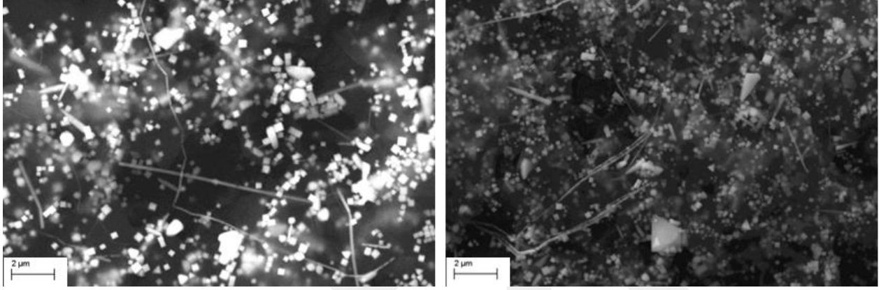
Şekil 47. 160 °C'de 48 saat bekletilen reaktörden elde ettiğimiz bakır nanotellere ait SEM görüntüleri
