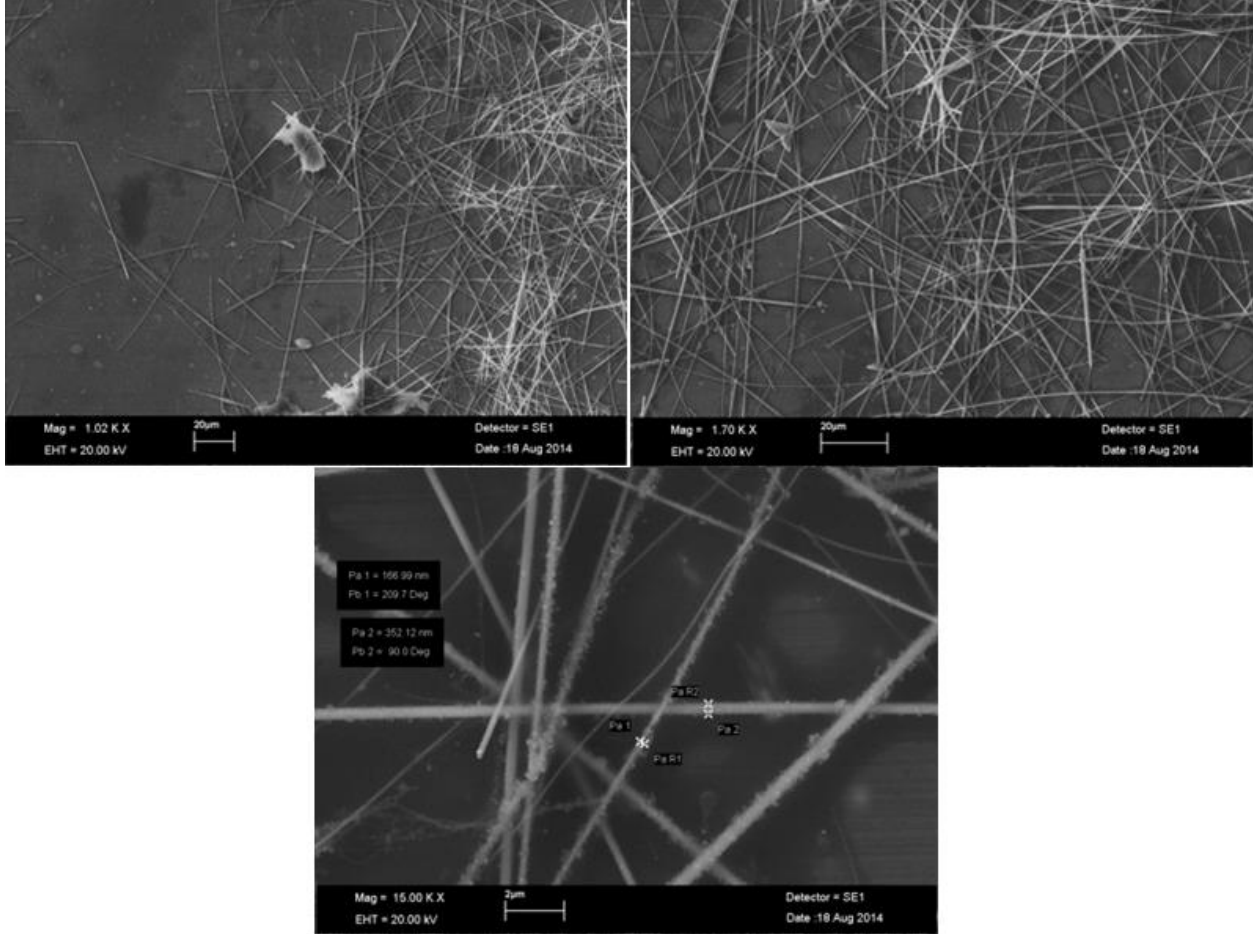
Şekil 23. \text{HAuCl}_4 kullanılarak iki fazlı titrasyonla Au kaplaması yapılmaya çalışılan bakır nanotellerin SEM görüntüleri.
