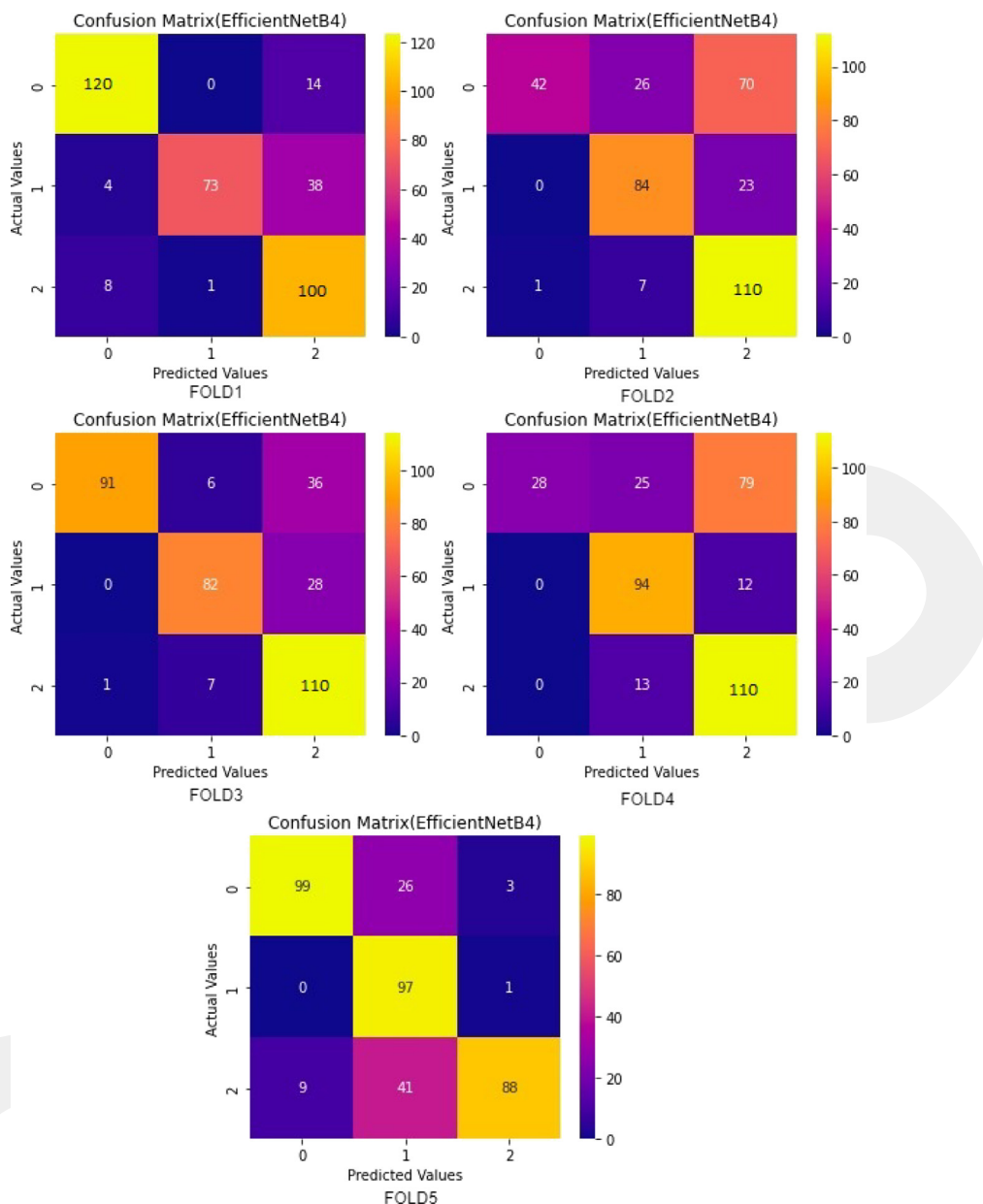
Fig. 6. Confusion Matrix:EfficientNetB4 on 5-Folds(0-Normal, 1-COVID19,2-Viral).
