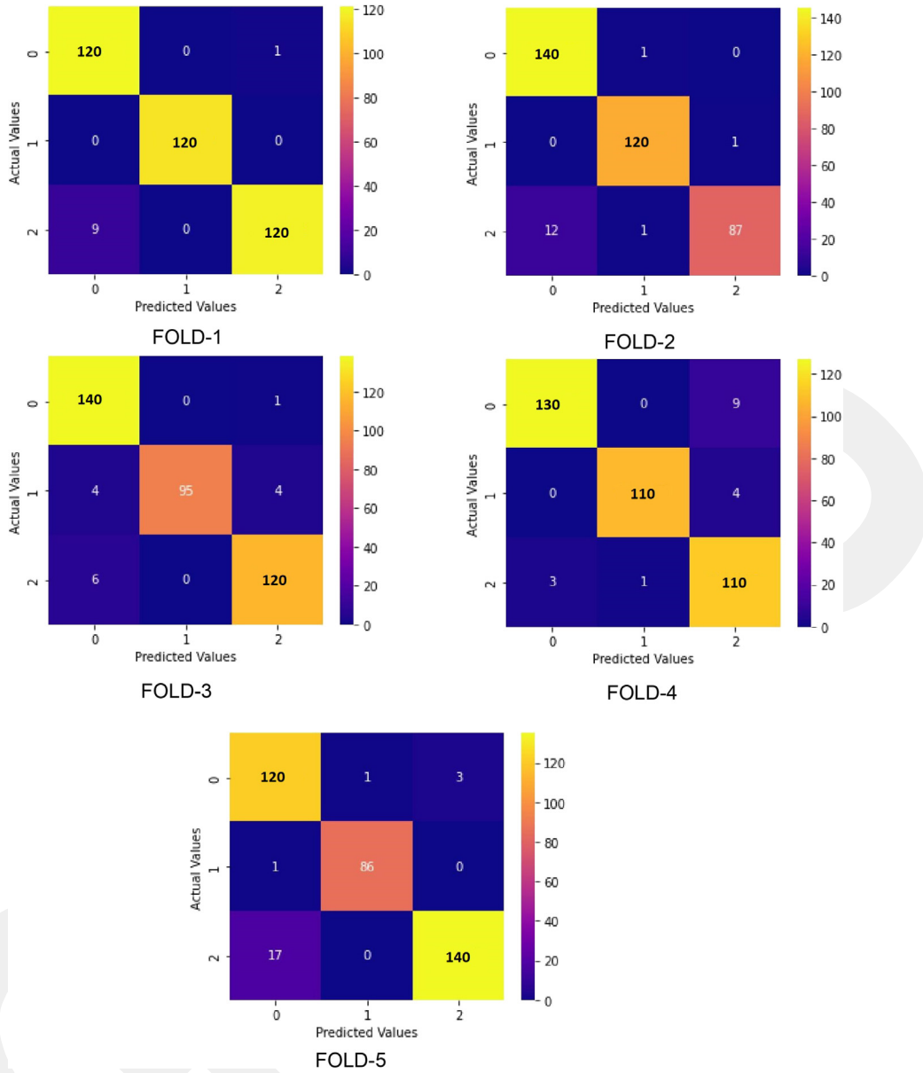
Fig. 4. Confusion Matrix:DenseNet121 on 5-Folds(0-Normal, 1-COVID19,2-Viral).
