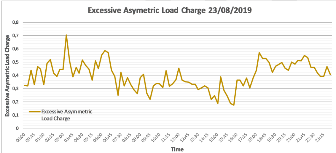
Şekil 4.25. Aşırı asimetrik yük şarjı
