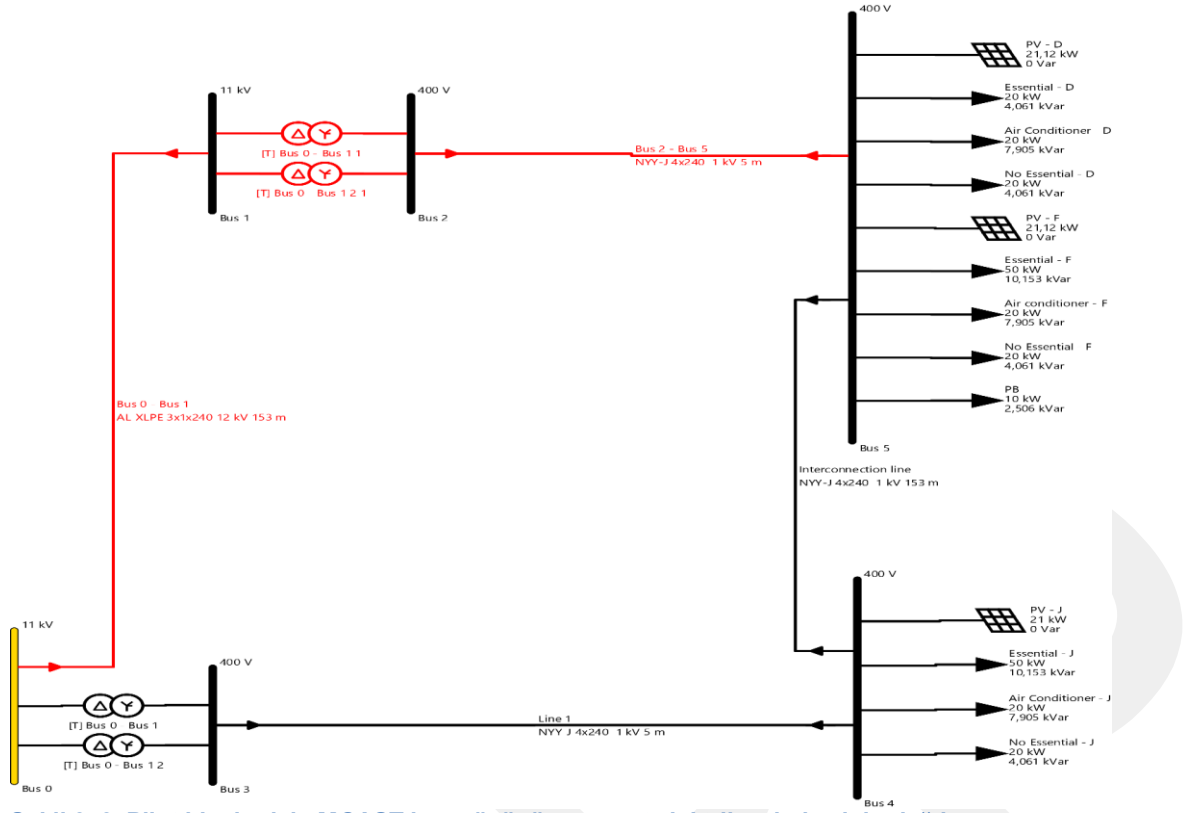
Şekil 3. 3. Pilot binalar için MCAST kampüsünün mevcut elektrik şebekesinin dağılımı
