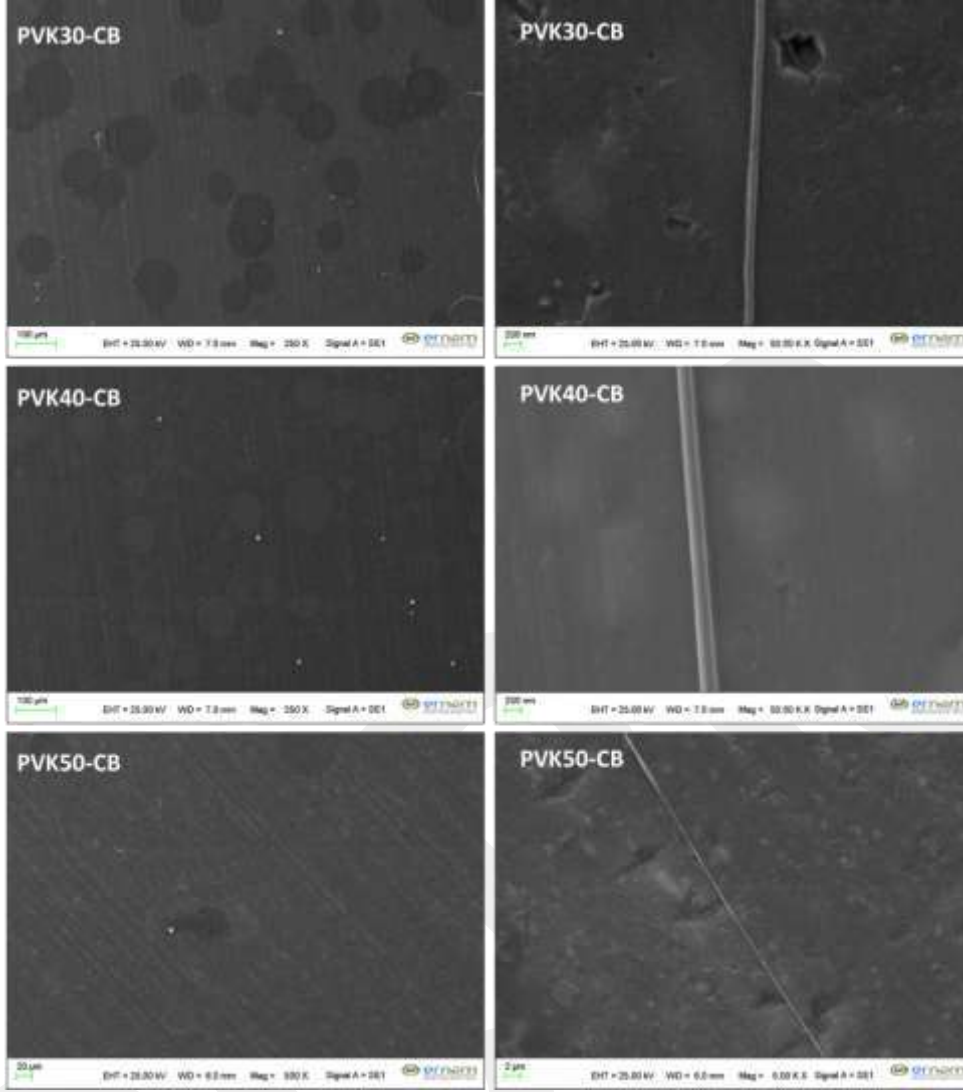
Şekil 52. PVK30-40-50-CB/DCM elektrospin yapılarının SEM görüntüleri
