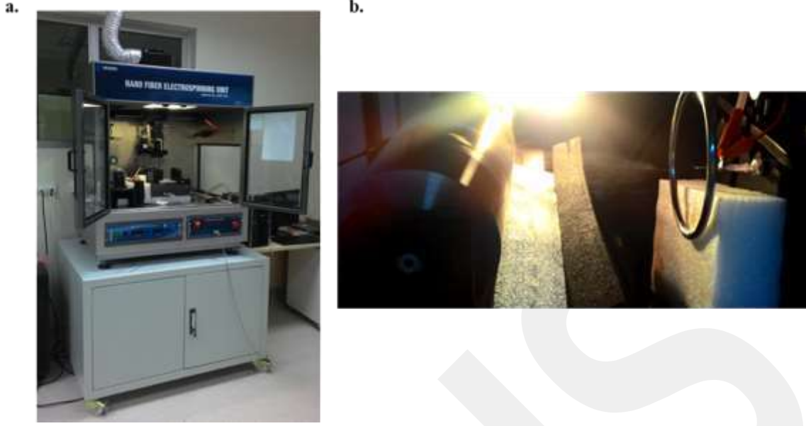
Şekil 30. Proje çalışmalarında kullanılan elektrospınleme sistemi. a) ünitenin dıştan görüntüsü, b) ünitenin elektrospınleme prosesi sırasındaki yakından çekilmiş görüntüsü
