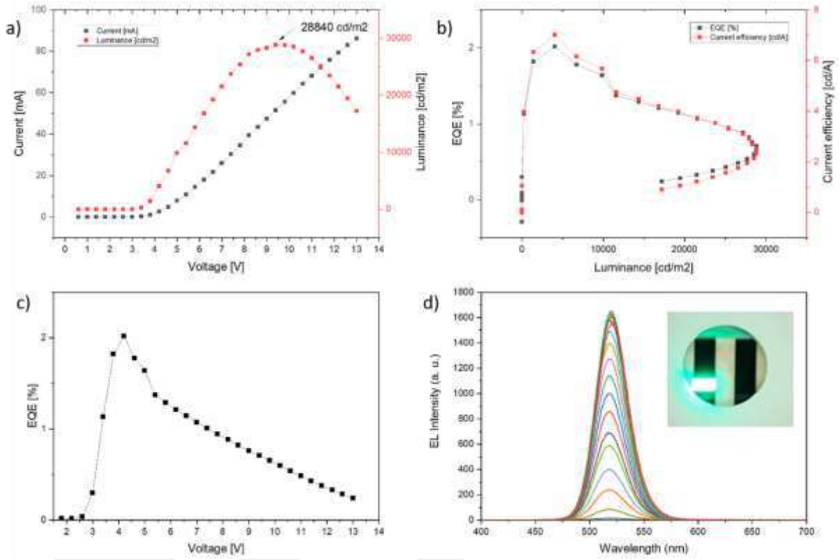
Şekil 61. Enkapsüle edilmiş QLED ölçüm grafikleri. a) I-V ve Voltaj-Lüminans ( \text{cd/m}^2 ), b) Lüminans ( \text{cd/m}^2 ) -EQE (kuantum verimliliği) ve Lüminans ( \text{cd/m}^2 ) – Akım verimliliği ( \text{cd/A} ) c) Voltaj-EQE, d) ışım spektrumu,
