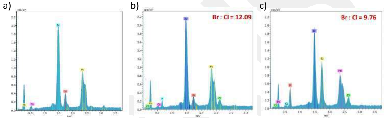
Şekil 107. a) Perovskit nanokristalin EDX analizi b) Floroalkilsilanın 10 saniye boyunca perovskit nanokristalin üzerine kaplandıktan sonraki EDX analizi c) Floroalkilsilanın 60 saniye boyunca perovskit nanokristalin üzerine kaplandıktan sonraki EDX analizi
