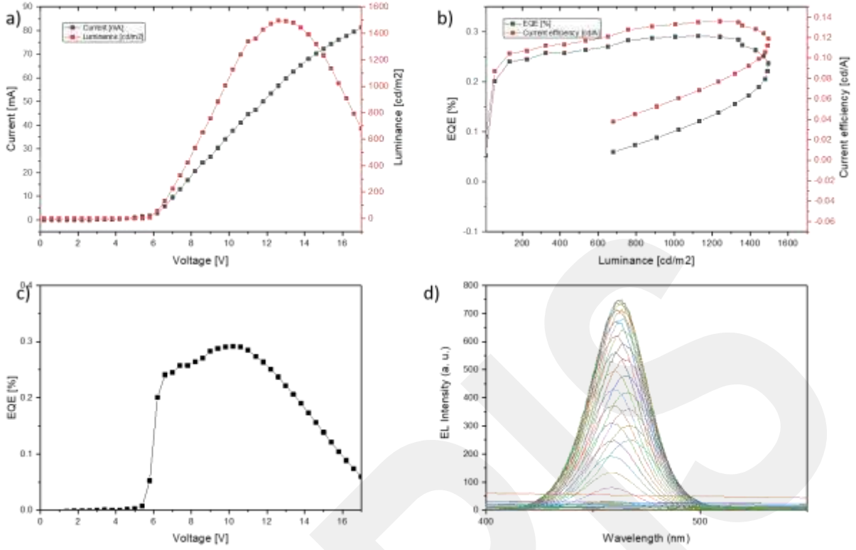
Şekil 64. Mavi QLED ölçüm sonuçları. a) I-V ve Voltaj-Lüminans (cd/m 2 ), b) Lüminans (cd/m 2 ) -EQE (kuantum verimliliği) ve Lüminans (cd/m 2 ) – Akım verimliliği (cd/A) c) Voltaj-EQE, d) ışım spektrumu
