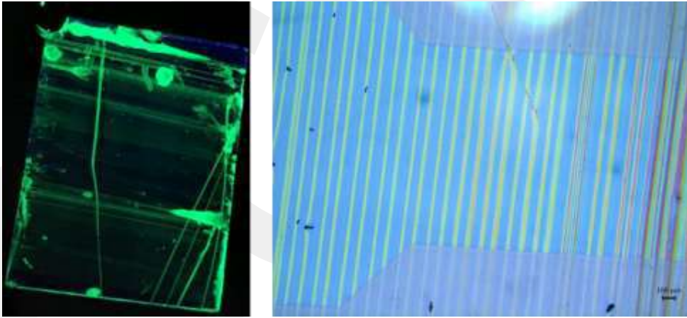
Şekil 81. YQD-PEO numunesinin görüntüleri. Sol: Fiber dizileri oluşturulmuş QLED altlığının UV ışığı altındaki fotoğrafı, sağ: QLED aktif hücre üzerine 100 µm aralıklarla yazılmış fiber dizilerinin optik mikroskop görüntüsü.
