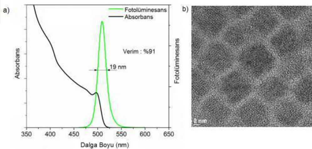
Şekil 73. Cs bazlı yeşil ışıyan PNC'ler a) absorbans ve fotoluminesans grafiđi b) HR-TEM görüntüsü
