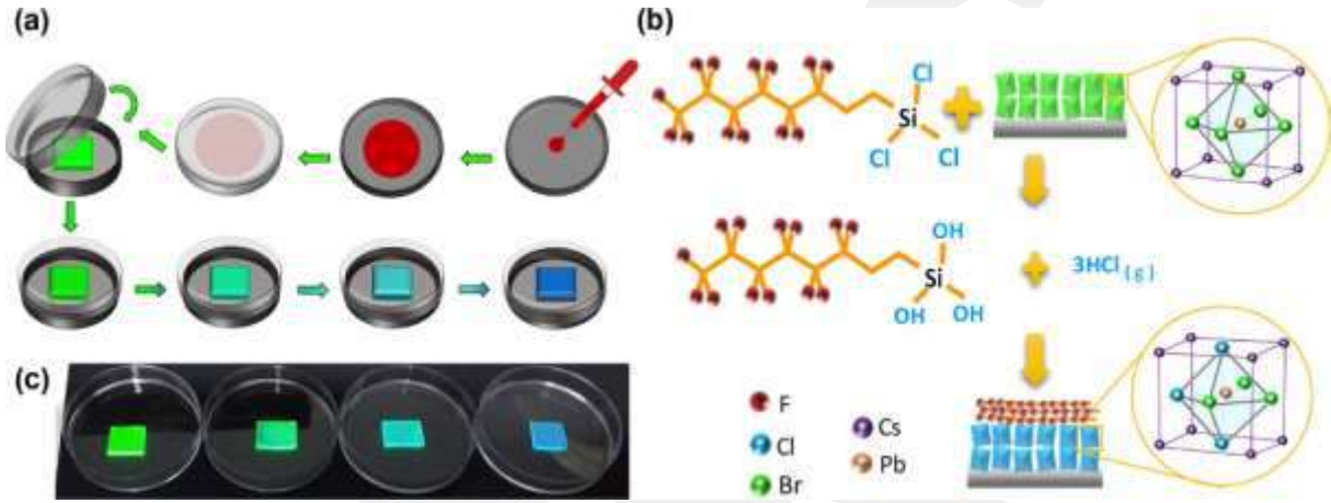
Şekil 104. Perovskit nanokristallerin kapsüllemesi a) Şematik gösterim b) Perovskit nanokristallerin ve floroalkilsilanın (Tridecafluoroalkyl-1,1,2,2-tetrahydrooctyltrichlorosilane) kimyasal ve kristal yapılarının gösterimi c) Artan süreye bağlı olarak floroalkilsilan buharına maruz kalan perovskit nanokristallerin renk değişimi.
