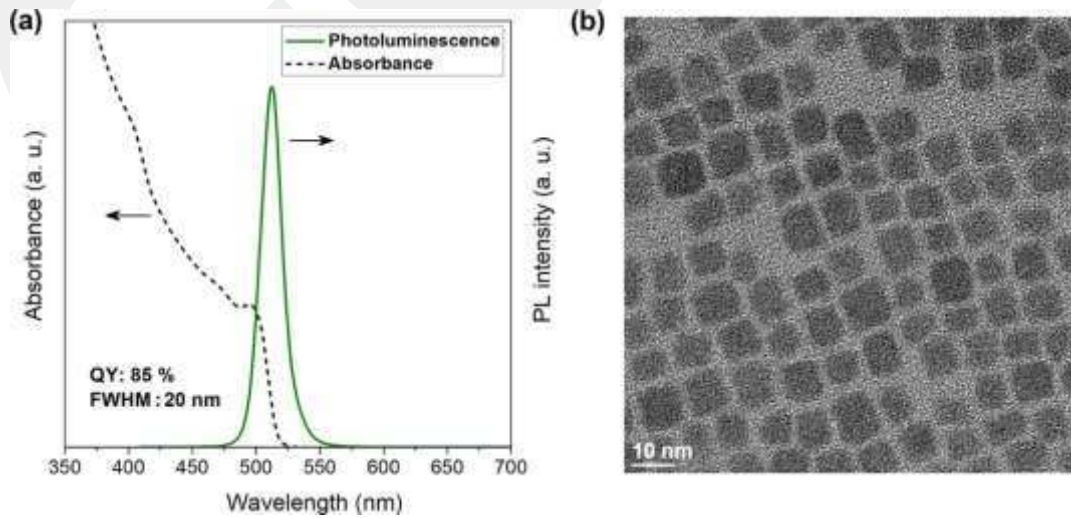
Şekil 105. a) Fotoluminesans ve absorpsiyon spektrumları b) Sentezlenen perovskit nanokristallerin TEM görüntüsü
