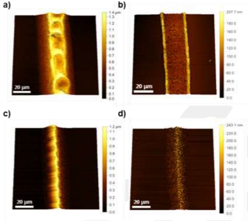
Şekil 76. Hareketli tabla hızının ve yüzey modifikasyonlarının desen boyut ve morfolojisine etkisi. a-b) Temiz silikon üzerindeki AFM görüntüleri c,d) hidrofobik alütaş üzerine sırasıyla 0,20 mm/s, 3,2 mm/s hızlarında dizilimini gösteren AFM görüntüleri
