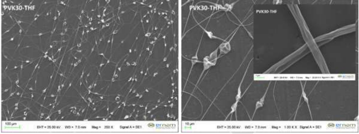
Şekil 49. PVK30-THF elektrospün yapılarının SEM görüntüleri
