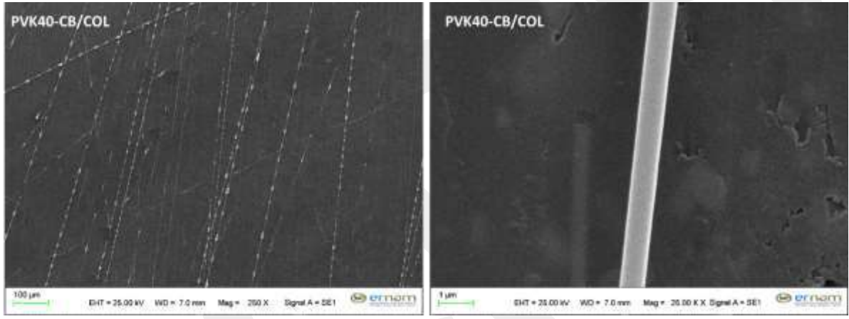
Şekil 50. PVK40-CB/COL elektrospün yapılarının SEM görüntüleri
