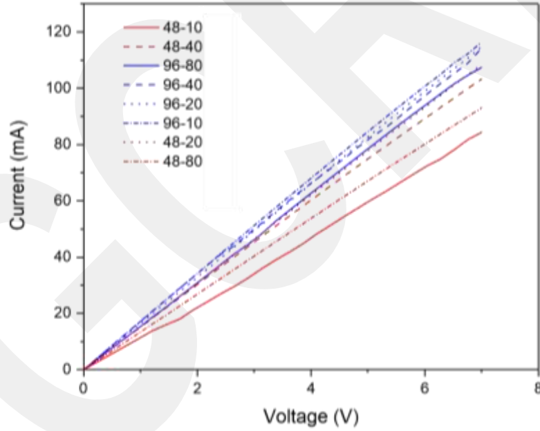
Şekil 43. Hole iletim katmanı olarak PVK-QD nanofiberleri içeren QLEDlerin elektriksel karakteristikleri
