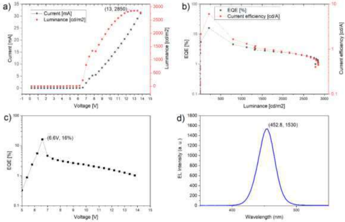
Şekil 69. Mavi ışık veren QLED aygıtının a) akım-voltaj ve parlaklık b) dış kuantum verimlilik c) voltaja bağlı dış kuantum verimlilik değişimi d) ışımaya spektrumu
