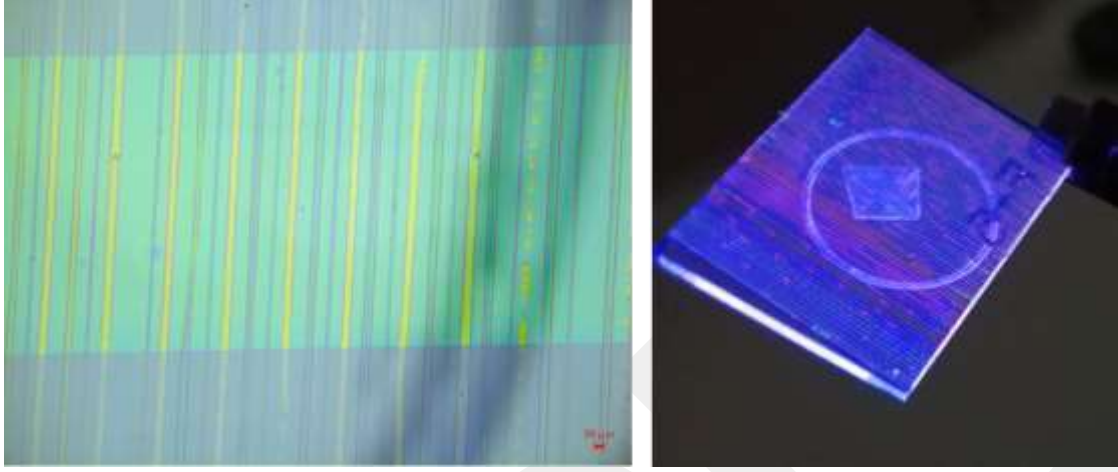
Şekil 85. Mavi, yeşil ve kırmızı kuantum noktacıkları barındıran bağımsız fiberlerin aynı yüzey üzerinde üretiminin gösterimi. Sol: QLED alttaşı üzerine sırasıyla 100 µm aralıklarla çizilmiş mavi, yeşil ve kırmızı kuantum nokta içeren fiber dizilerinin optik görüntüsü, Sağ: Fiber dizileri oluşturulmuş QLED altlığının UV ışığı altındaki fotoğrafı
