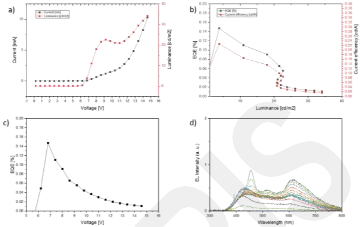
Şekil 95. Kuantum noktacıkların birbirine karıştırılarak çizilen fiberlerin ışıyan katmanda bulunduğu beyaz QLED'in a) I-V ve Voltaj-Lüminans ( \text{cd/m}^2 ), b) Lüminans ( \text{cd/m}^2 ) -EQE (kuantum verimliliği) ve Lüminans ( \text{cd/m}^2 ) – Akım verimliliği ( \text{cd/A} ) c) Voltaj-EQE, d) ışımaya spektrumu
