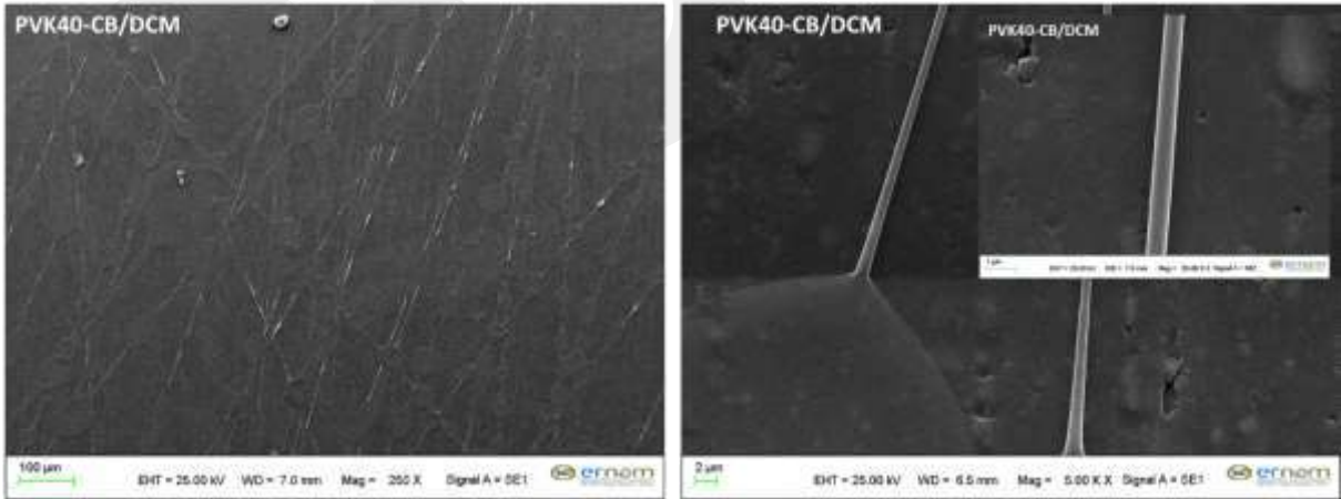
Şekil 51. PVK40-CB/DCM elektrospün yapılarının SEM görüntüleri
