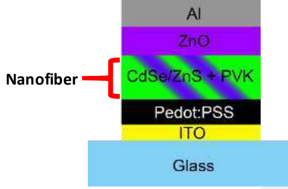
Şekil 42. Kuantum noktacıların hole iletim katmanı olarak PVK nanofiberleri içerisinde olduğu QLED yapısı.
