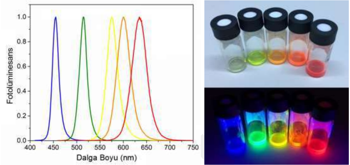
Şekil 72. Anyon değişimi ile yeşil ışıyan PNC'lerden elde edilmiş farklı renkteki kuantum noktacıklara ait ışıma grafiđi ve UV ışığı altındaki görüntüleri
