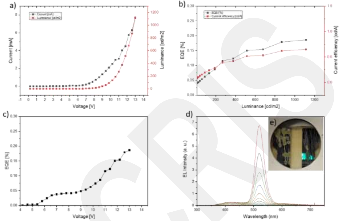
Şekil 87. Polimer kullanılmadan sadece kuantum noktacık kullanılarak üretilen fiber QLED'in a) I-V ve Voltaj-Lüminans (cd/m 2 ), b) Lüminans (cd/m 2 )-EQE (kuantum verimliliği) ve Lüminans (cd/m 2 ) – Akım verimliliği (cd/A) c) Voltaj-EQE, d) ışımaya spektrumu, e) cihazın fotoğrafı
