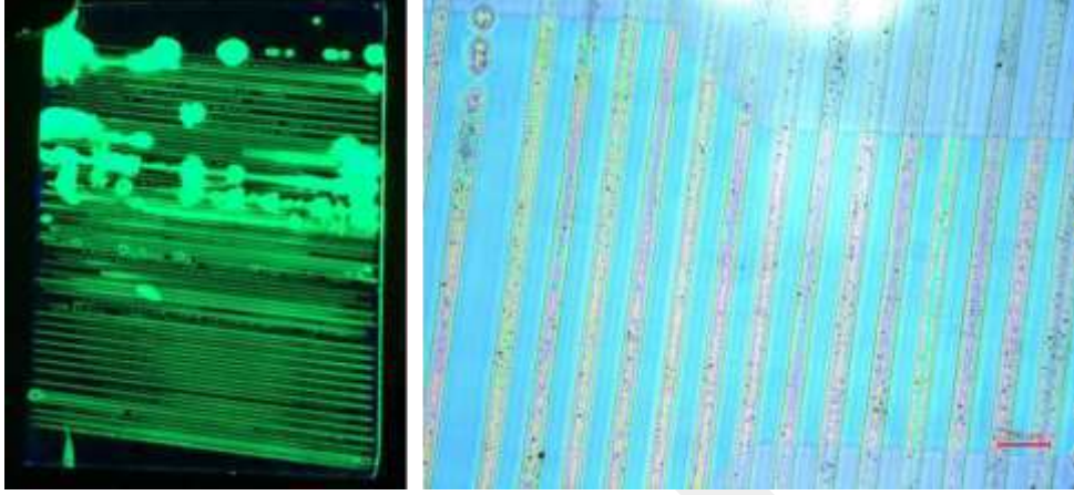
Şekil 80. YQD-PVK numunesinin görüntüleri. Sol: Fiber dizileri oluşturulmuş QLED altlığının UV ışığı altındaki fotoğrafı, sağ: QLED aktif hücre üzerine 100 µm aralıklarla yazılmış fiber dizilerinin optik mikroskop görüntüsü.
