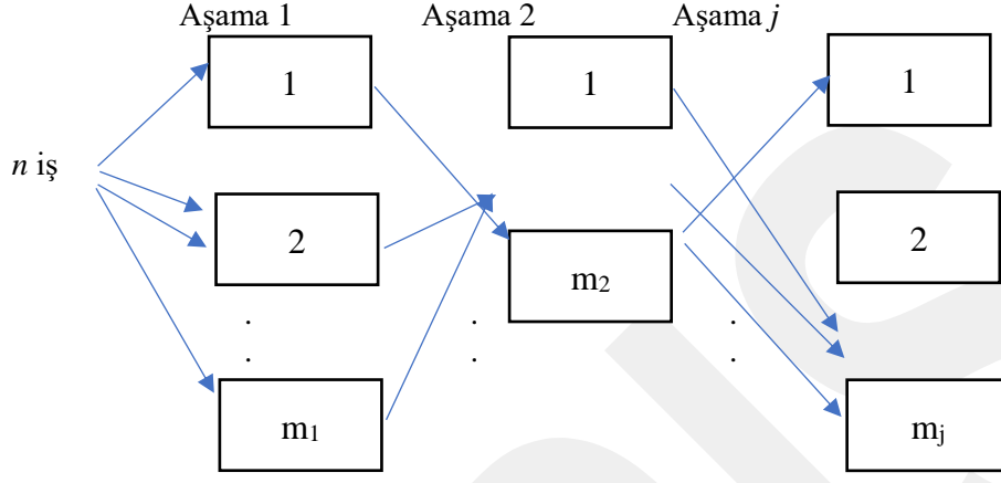
Şekil 1. Hibrit akış tipi üretim ortamı
