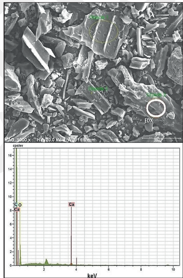
Şekil 4. Odun atığı SEM-EDX görüntüsü ve element pikleri
