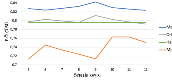
Şekil 3. Cleveland veri kümesi üzerinde, farklı sayıda öznelikler için, MLP sınıflandırıcısının Öznelik Seçimi Uygulanmadığındaki (ÖSU, Ham) ve topluluk öznelik seçimi kullanıldığında Maksimum (Max), Minimum (Min), Ortalama (Ort) F-Ölçüsü Değerleri
