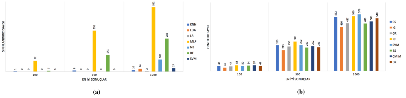
Şekil 2. Cleveland veri kümesinde F-Ölçüsü performans ölçütüne göre ilk 100, ilk 500 ve ilk 1000 en iyi modelde en sık kullanılan (a) sınıflandırma yöntemleri, (b) öznelik seçim yöntemleri.
