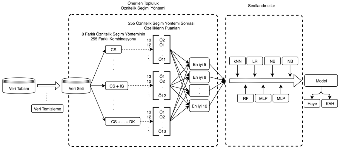
Şekil 1. Önerilen topluluk öz nitelik seçim yöntemi ve sınıflandırma işleminin genel gösterimi
