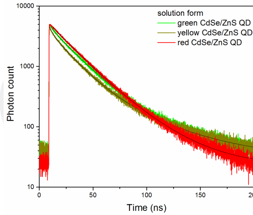
Şekil 73. CdSe/ZnS Yeşil, sarı ve kırmızı kuantum noktacıkların zaman çözünürlüklü fotoluminesans ölçümü.
