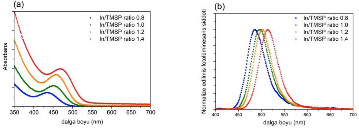
Şekil 13. (a) Absorbans değerinin, (b) fotoluminesans spektrumunun In/P miktarı ile değişimi Şekil 13 (a)'daki absorbans ve Şekil 13 (b)'deki fotoluminesans spektrumunda In/P oranı arttıkça dalga boyunun arttığını görmekteyiz.
