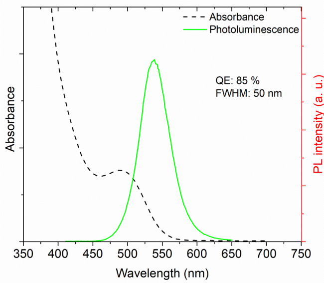
Şekil 48. Sentez sonucu elde edilen kuantum nokta yapıların absorban ve fotoluminesans spektrumları
