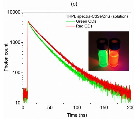
Şekil 77. (a) Kırmızı (b) yeşil ışıyan CdSe/ZnS kuantum noktacıklarının fotolüminesans, absorbans ve fotolüminesans uyarılma spektrumu (c) zaman çözünürlüklü fotolüminesans ölçümü
