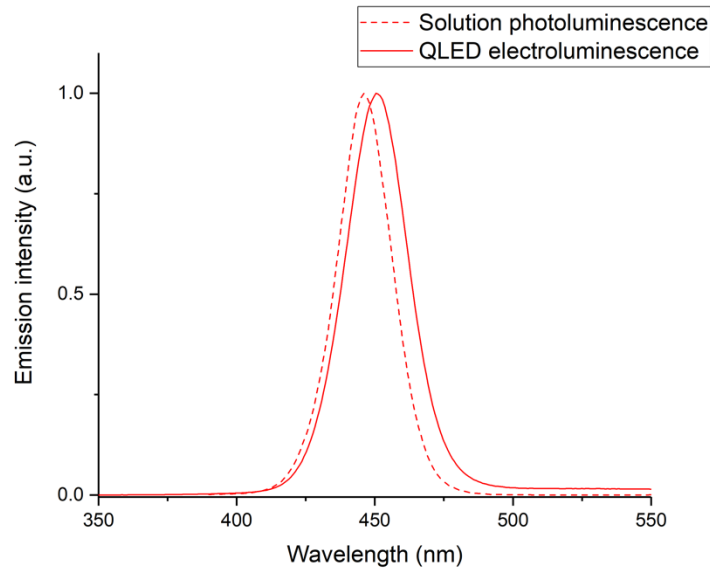
Şekil 106. 2 numaralı OLED cihazın elektrolüminesans spektrumu ile kullanılan kuantum noktacı solüsyon halindeki fotolüminesans spektrumunun kıyaslamalı grafiği
