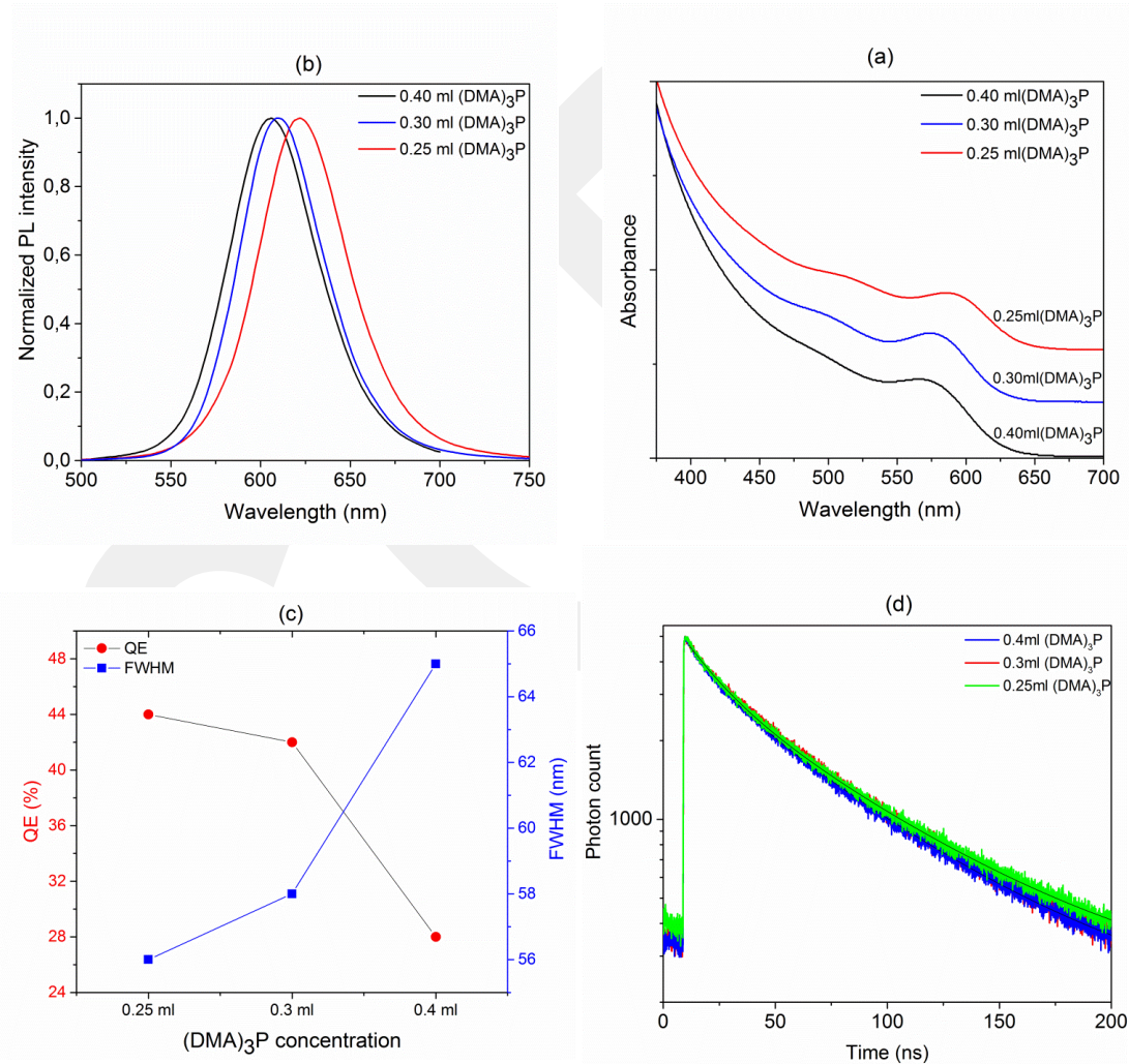
Şekil 35. Kullanılan (DMA) 3 P miktarının değişimi ile değişen (a) Absorbans (b) Fotolüminesans (c)Kuantum verimlilik-FWHM (d) Zaman çözünürlüklü fotolüminesans ölçümü
