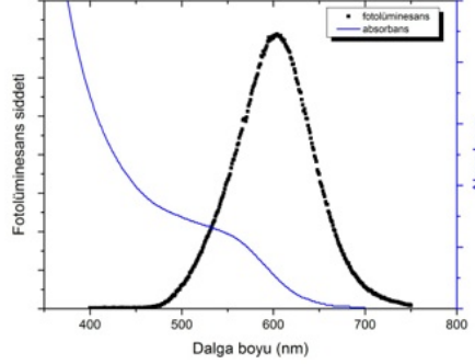
Şekil 46. Sentezlenen InP/GaP/ZnS için absorbands ve fotoluminesans spektrumu
