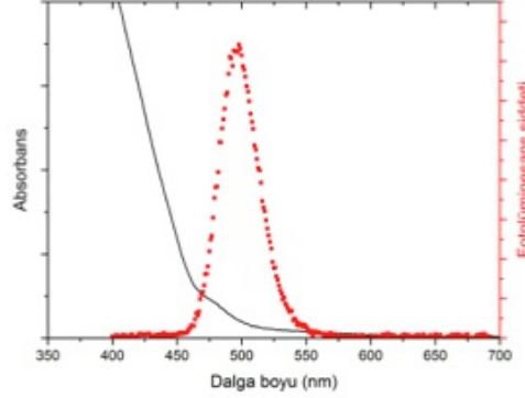
Şekil 66. Sentezlenen yeşil ışıyan CdSe/ZnS kuantum noktacıkların absorpsiyon ve fotolüminesans spektrumu
