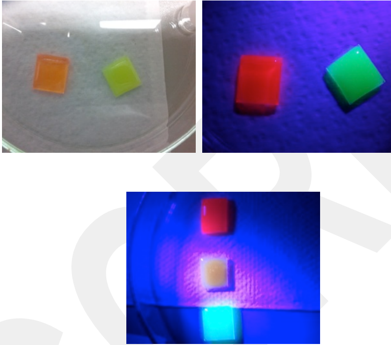
Şekil 74. Karışımın cam üzerine dökülmesinin hemen sonrasındaki fotoğraflardan a) Yeşil ve kırmızı film-gün ışığında b) Yeşil ve kırmızı film-UV ışığındaki görüntüsü c) yeşil, sarı ve kırmızı kuantum nokta polimer filmlerin cam üzerine döküldükten hemen sonraki fotoğrafı
