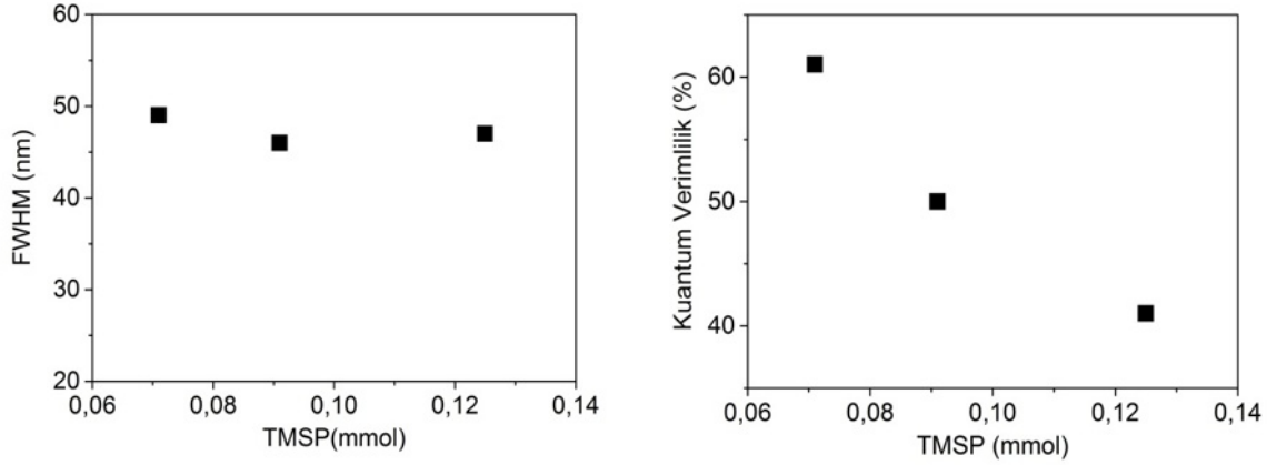
Şekil 11. Kuantum verimliliğin ve FWHM değerinin (TMS) 3 P miktarı ile değişimi
