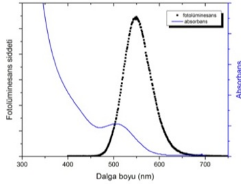
Şekil 47. Palmitik asit miktarı modifiye edilerek sentezlenen InP/GaP/ZnS için absorbands ve fotoluminesans spektrumu
