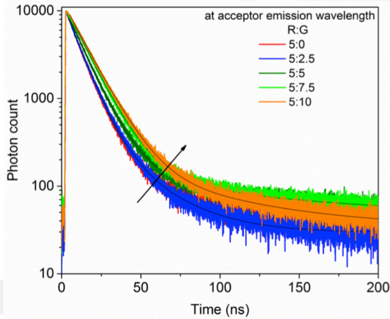
Şekil 81. (Donor/akseptör oranlarının değişimine göre) Akseptör şıma dalgaboyunda alınan zaman çözünürlüklü fotoluminesans ölçümü (akseptör ışıma dalgaboyunda)
