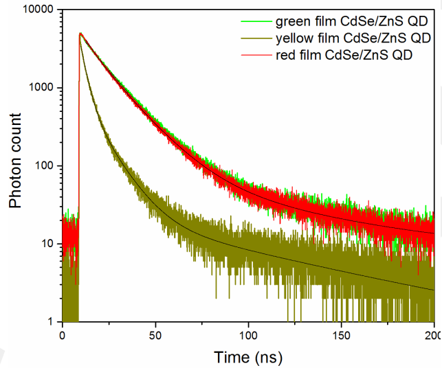
Şekil 76. Yeşil, sarı ve kırmızı filmlerin zaman çözünürlüklü fotoluminesans eğrileri
