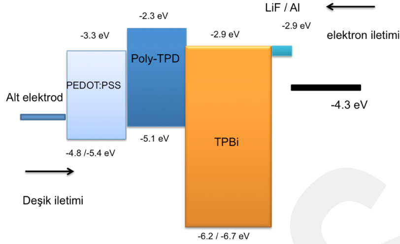
Şekil 3. Mavi ışık saçan örnek Alt elektrot/PEDOT:PSS/Poly-TPD/TPBi/LiF/Al aygıt mimarileri ve yaklaşık temsili HOMO-LUMO seviyelerine uygun bant diyagram gösterimi
