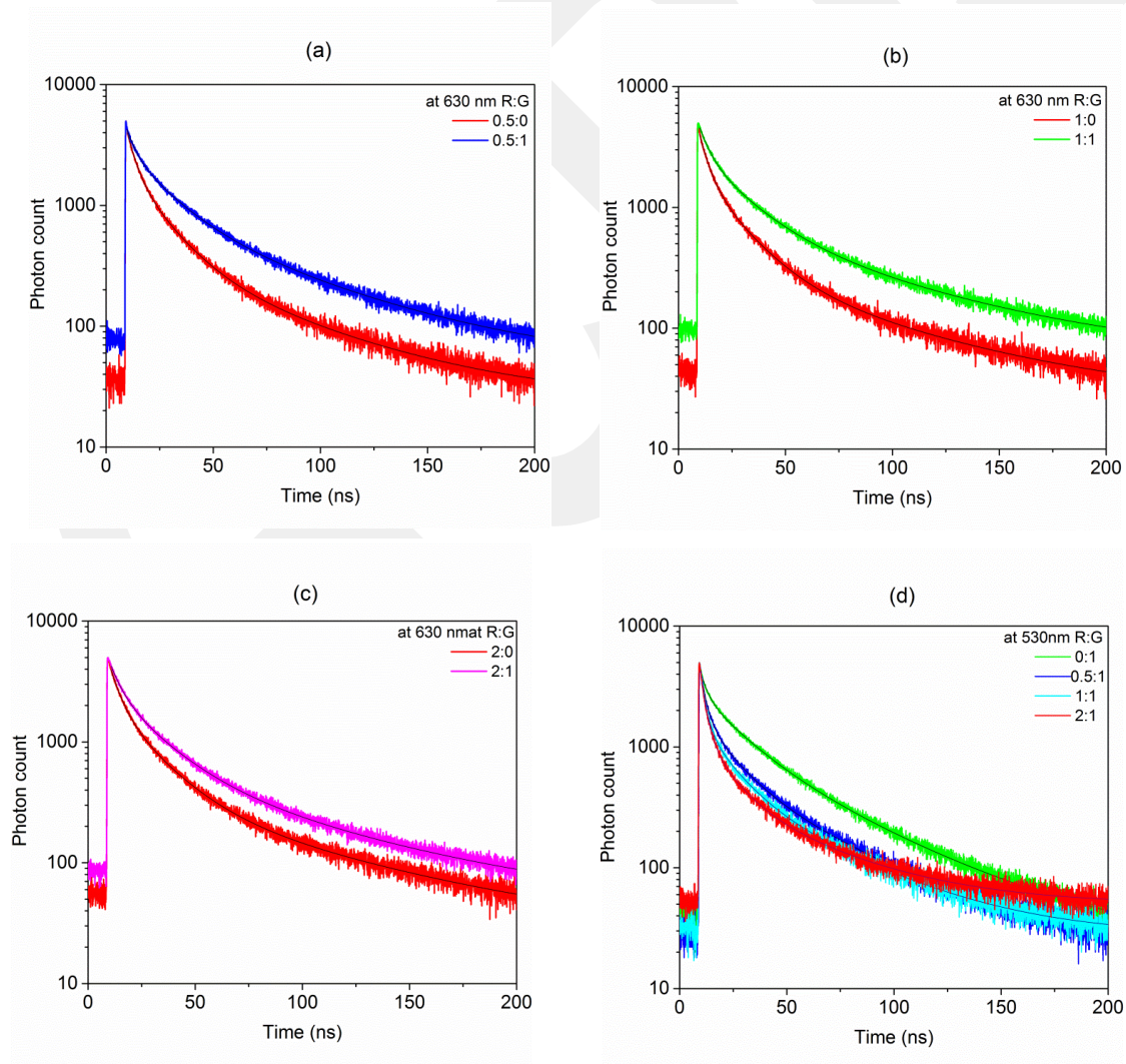
Şekil 38. Farklı konsantrasyonlarda hazırlanan polimerik kuantum noktacıklı filmlerin zaman çözünürlüklü fotoluminesans ölçümü.
