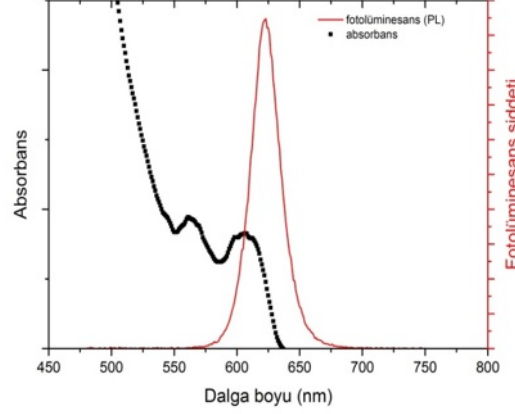
Şekil 65. 90 saniye beklenilerek sentezlenen kuantum parçacıkların absorpsiyon ve fotoluminesans spektrumu
