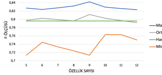
Şekil 3. Cleveland veri kümesi üzerinde, farklı sayıda öznelikler için, MLP sınıflandırıcısının Öznelik Seçimi Uygulanmadığındaki (ÖSU, Ham) ve topluluk öznelik seçimi kullanıldığındaki Maksimum (Max), Minimum (Min), Ortalama (Ort) F-Ölçüsü Değerleri
